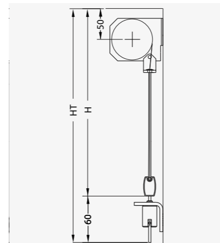
Guidage câbles
