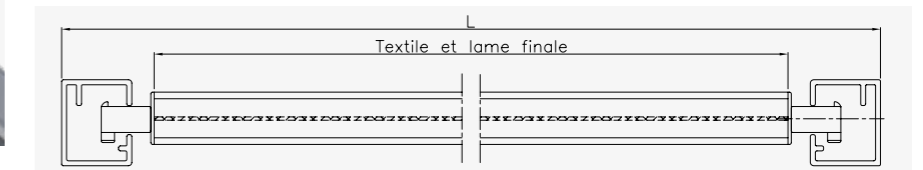
Exécution Soloscreen® III Box Fix
