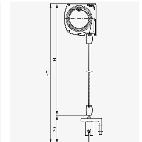
Guidage câbles
