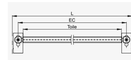
Guidage câbles
